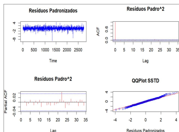
Figura 5. Análise dos resíduos do modelo GARCH (1,1).
